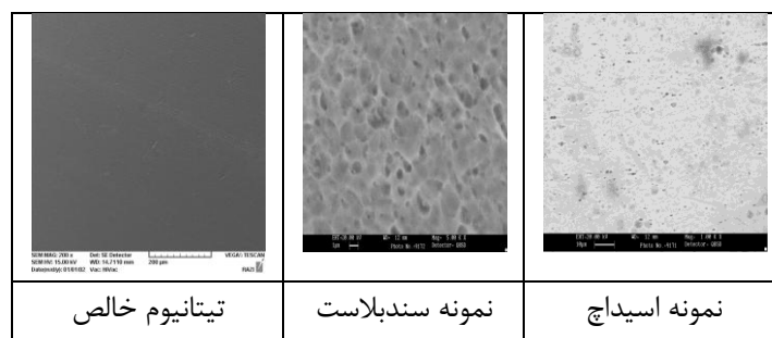
شکل ۱- نمونه وایر های مورد آزمایش پس از آماده سازی سطحی. میکروسکوپ الکترونی (SEM) بزرگنمایی \times 1000
